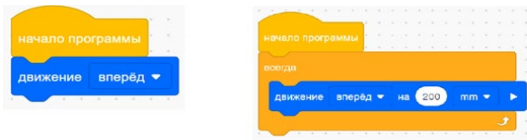
Рис. 29. Аналог бесконечного цикла
